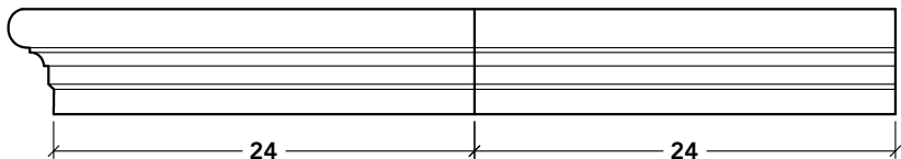
S-35
