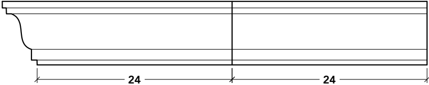
S-15
