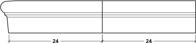
S-41
